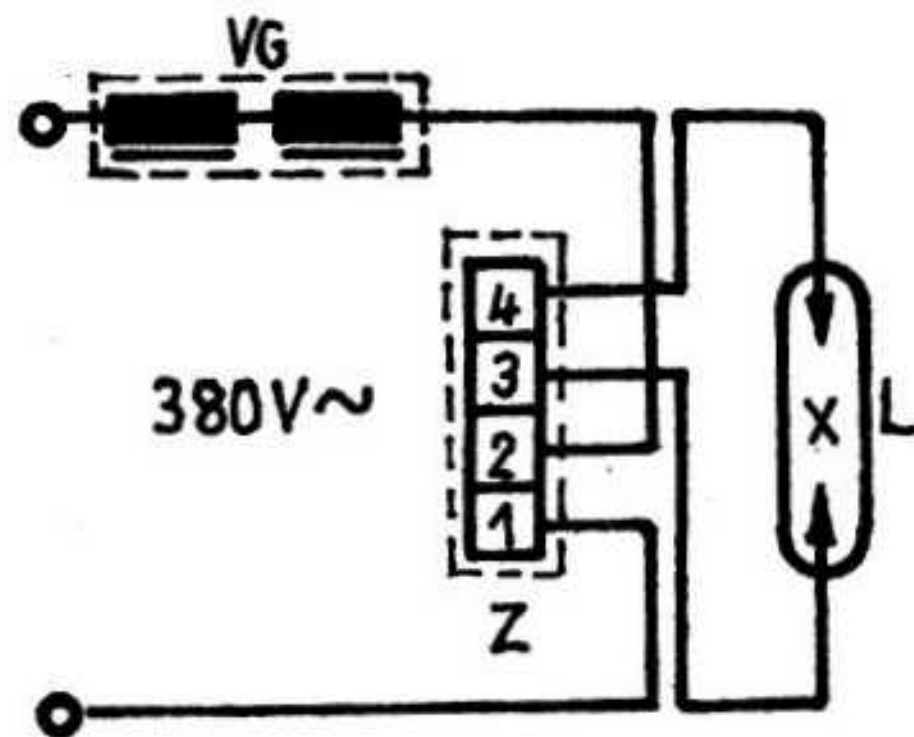
Schaltbild 2
