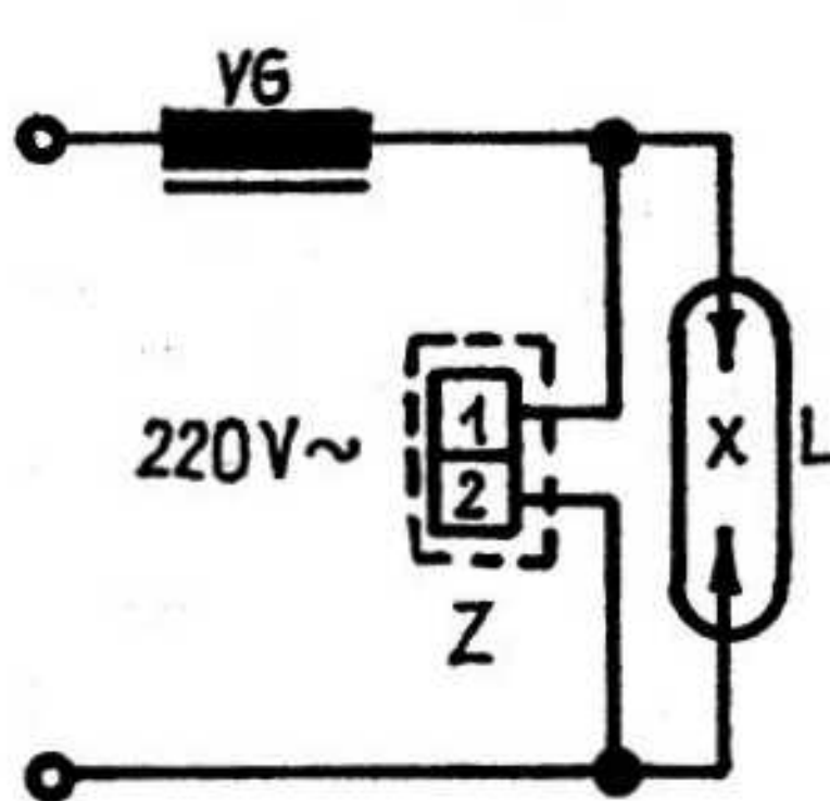
Schaltbild 1
