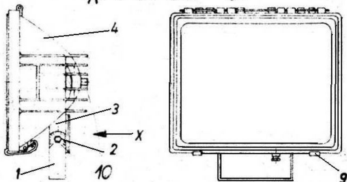
Ansicht X
